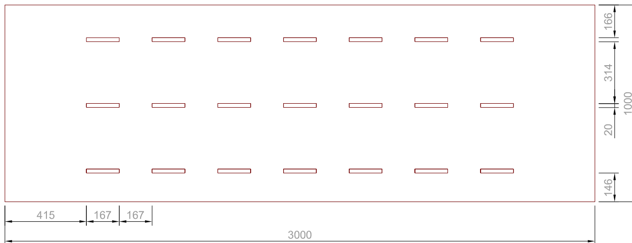
Bovenaanzicht
