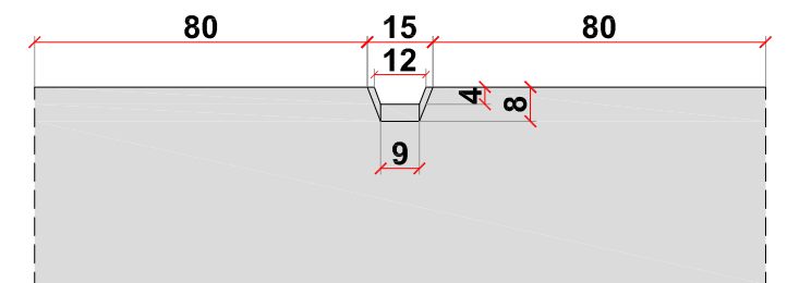
DETAIL C: LANGSGLEUF (SCHAAL 1:2)
