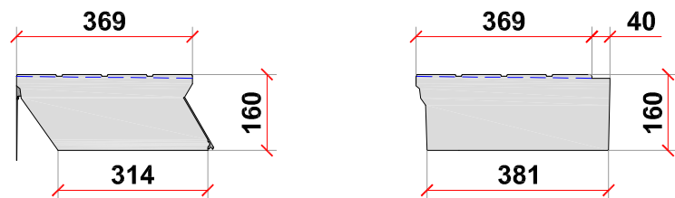
ZIJAANZICHT
