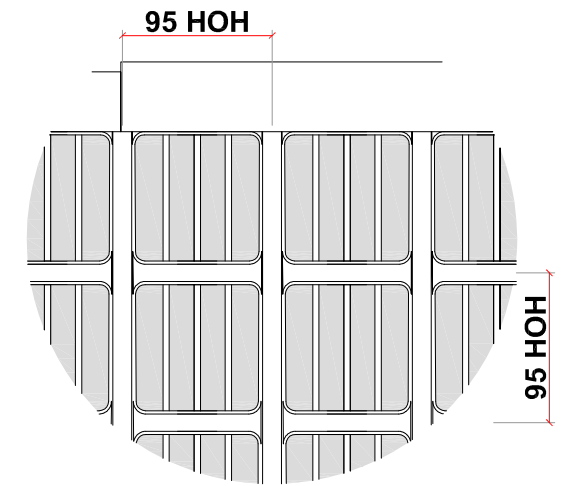
DETAIL A: TEGELMOTIEF MET PROFIEL (SCHAAL 1:5)
