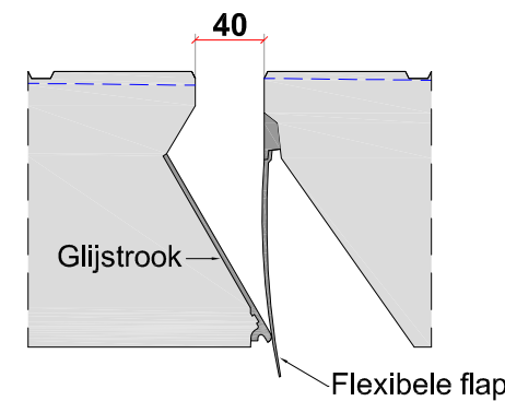
DETAIL MESTSLEUF (SCHAAL 1:5)
