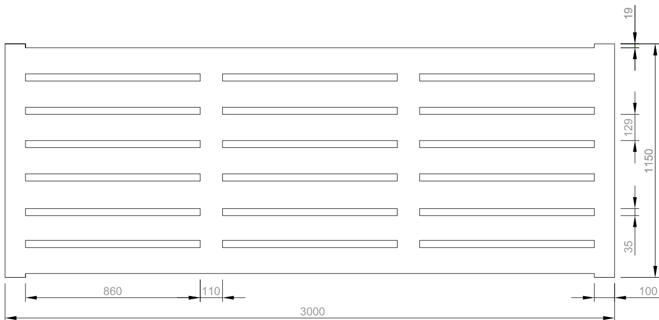
Bovenaanzicht
