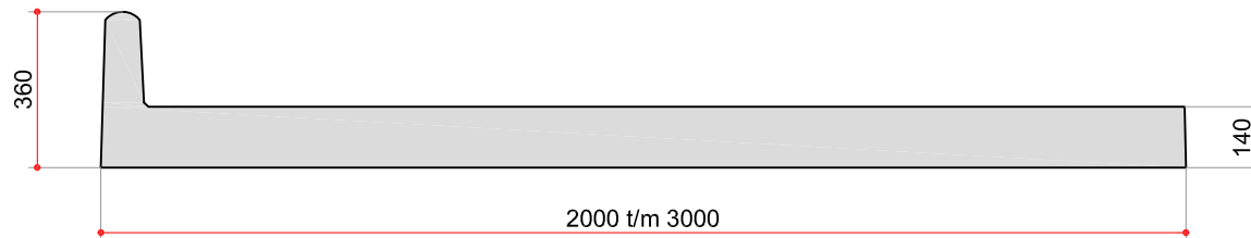
Lengtedoorsnede
