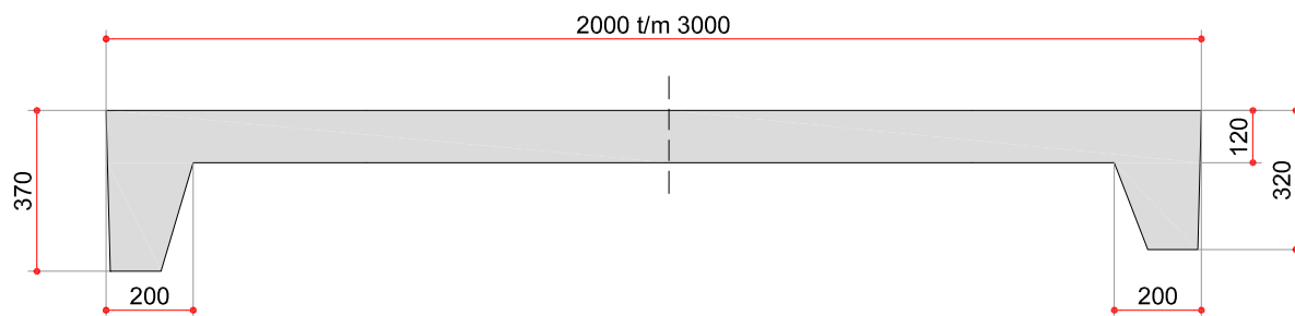
Lengtedoorsnede
